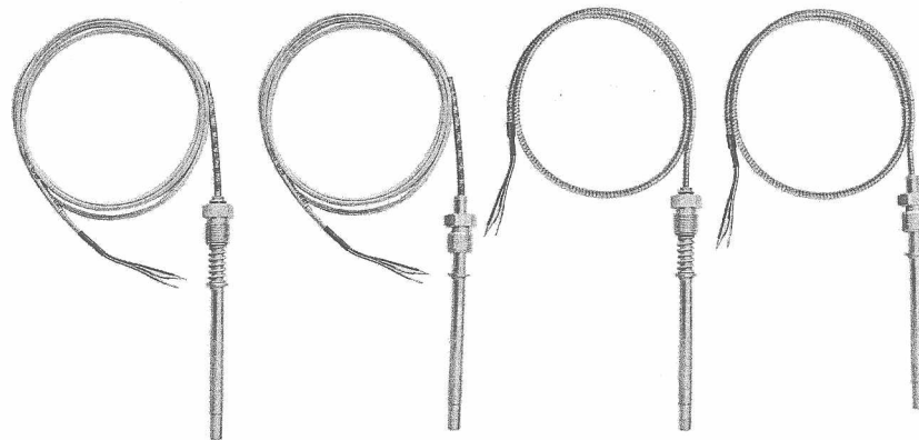
Рис.3 Общепромышленные ТСМ 321М-Оп, ТСП 321М-Оп и взрывозащищенные ТСМ 321М-Exi, ТСП 321М-Exi
