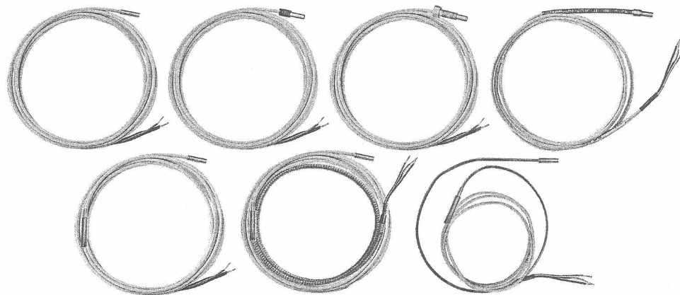
Рис.1 Общепромышленные ТСМ 319М-Оп, ТСП 319М-Оп и взрывозащищенные ТСМ 319М-Ехi, ТСП 319М-Ехi
