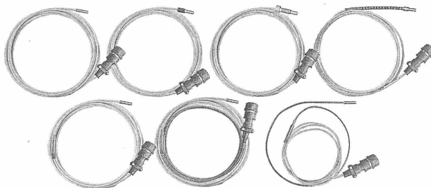
Рис.5 Общепромышленные ТСМ 323М-Оп, ТСП 323М-Оп и взрывозащищенные ТСМ 323М-Ехi, ТСП 323М-Ехi
