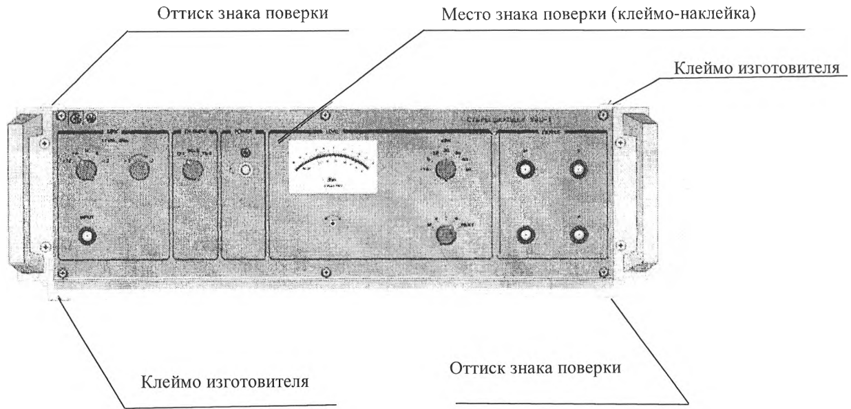
Рисунок А.1 – Вид измерителя спереди
