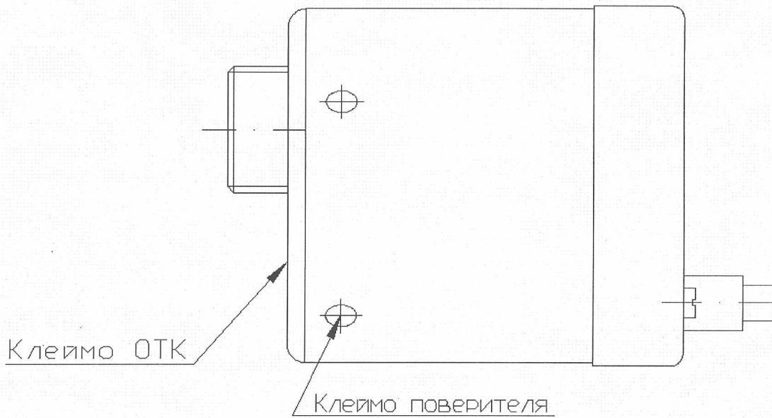
Рисунок А.2 – Схема клеймения вольтамперметра ВА-040
