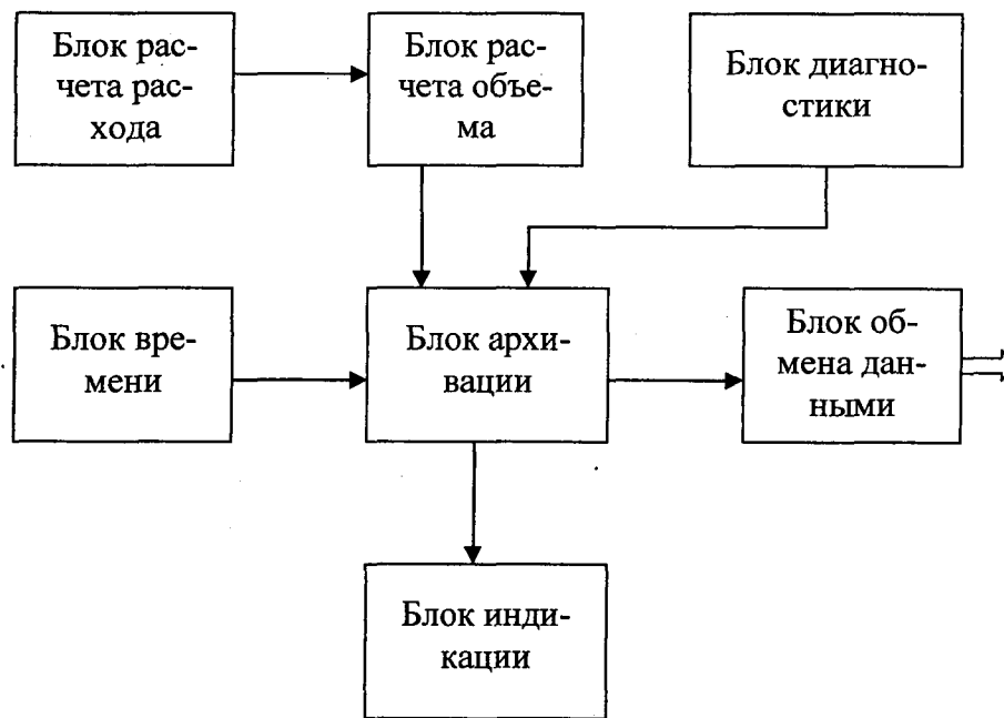
Рис. 3. Структура ПО
