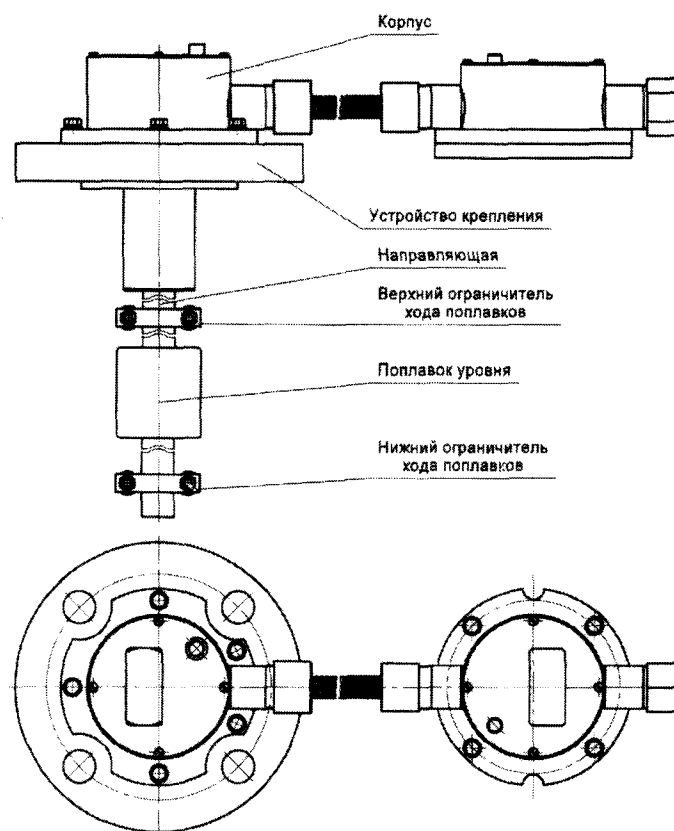
Рисунок 5 – Общий вид преобразователя ПМП-118-2ПИ-3В
