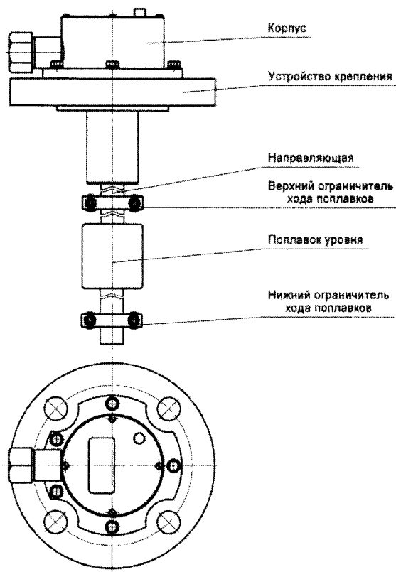
Рисунок 4 – Общий вид преобразователя ПМП-118-ВЦ
