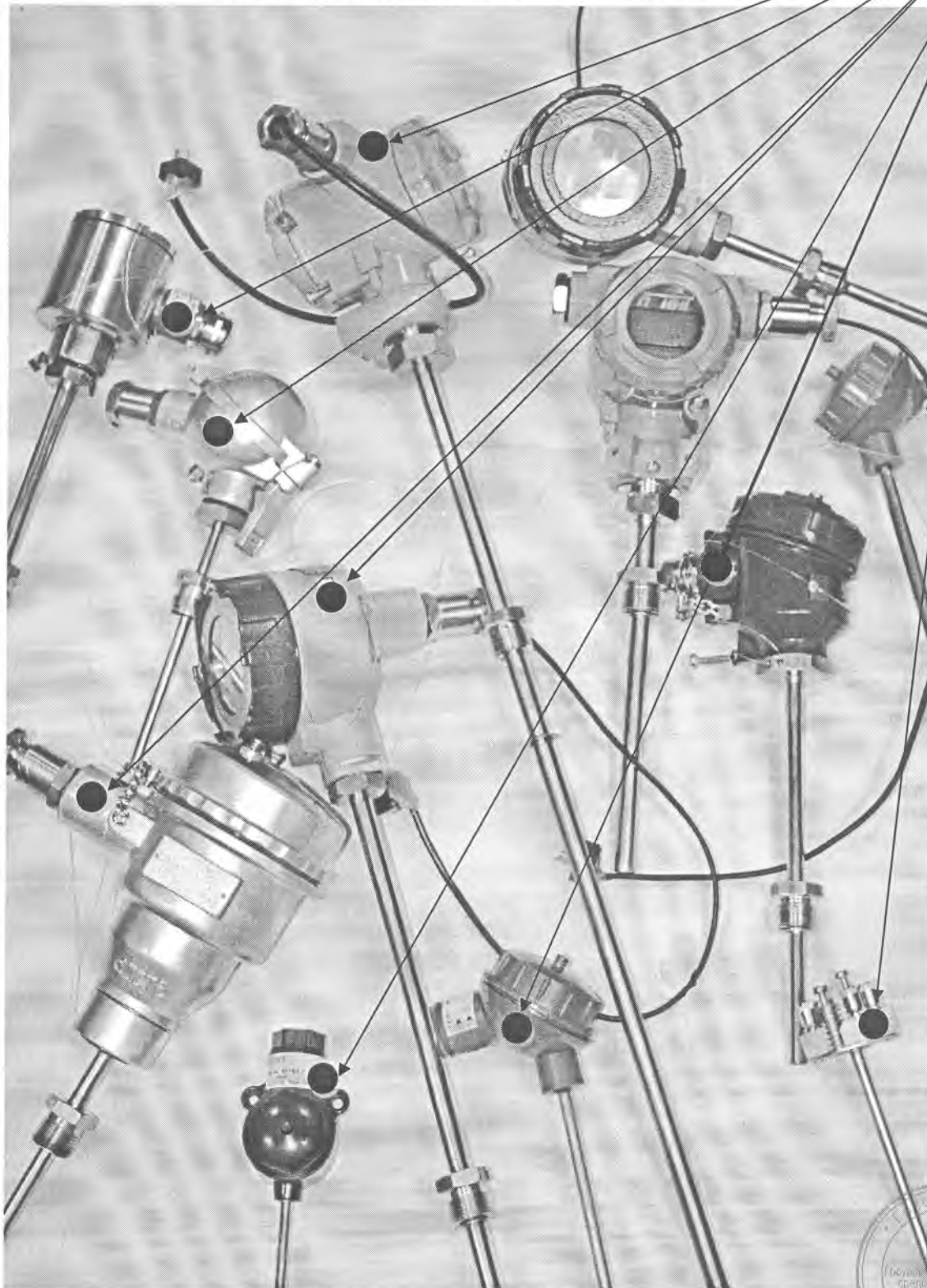
Рисунок А.1 - Внешний вид термопреобразователей сопротивления ТС-Б и место нанесения знака поверки в виде клейма-наклейки.
