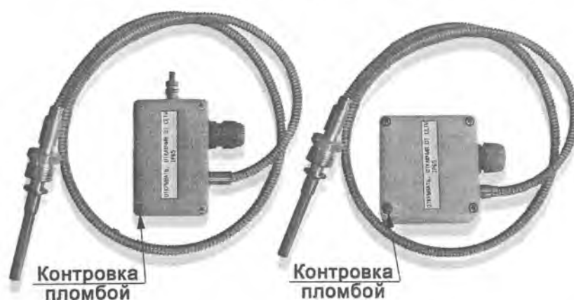
Погружаемые термопреобразователи с соединительным кабелем с видом взрывозащиты «Искробезопасная электрическая цепь» по ГОСТ Р 51330.10-99
