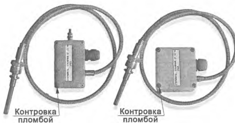
Погружаемые ППТ моделей ППТСК (с соединительным кабелем) с видом взрывозащиты «Искробезопасная электрическая цепь «i» по ГОСТ Р 52350.11-2005
