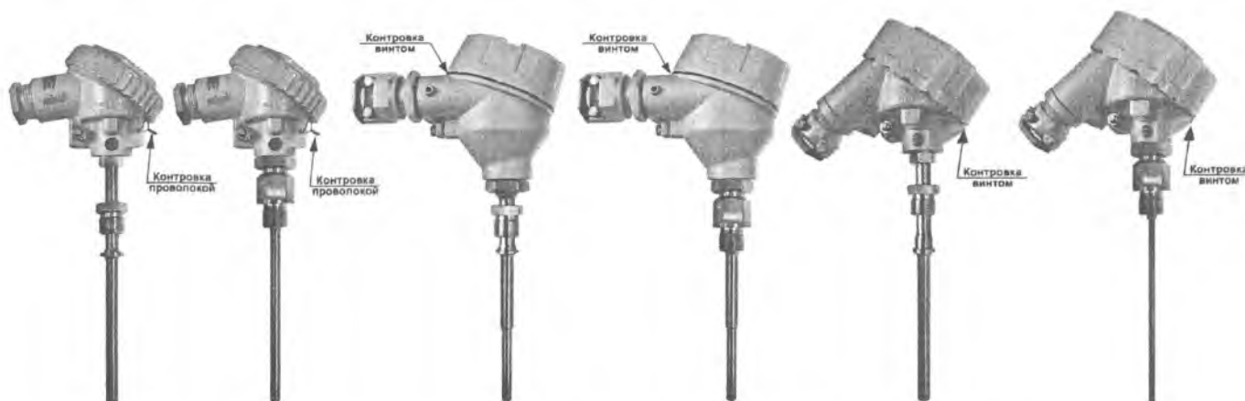
Погружаемые ППТ моделей ППТС/С, ППТС/В, ППТС/ОВ с видом взрывозащиты «Искробезопасная электрическая цепь «i» по ГОСТ Р 52350.11-2005
