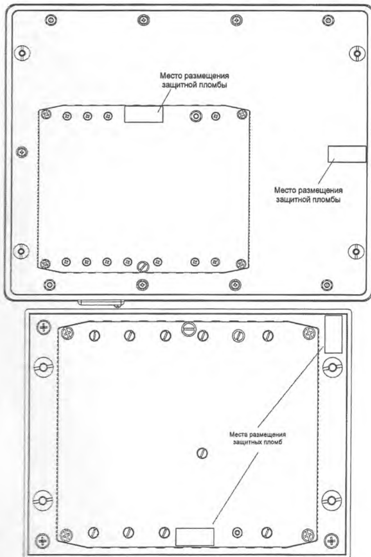
Рисунок 2 – Схема и внешний вид пломбировки регистратора от несанкционированного доступа.
