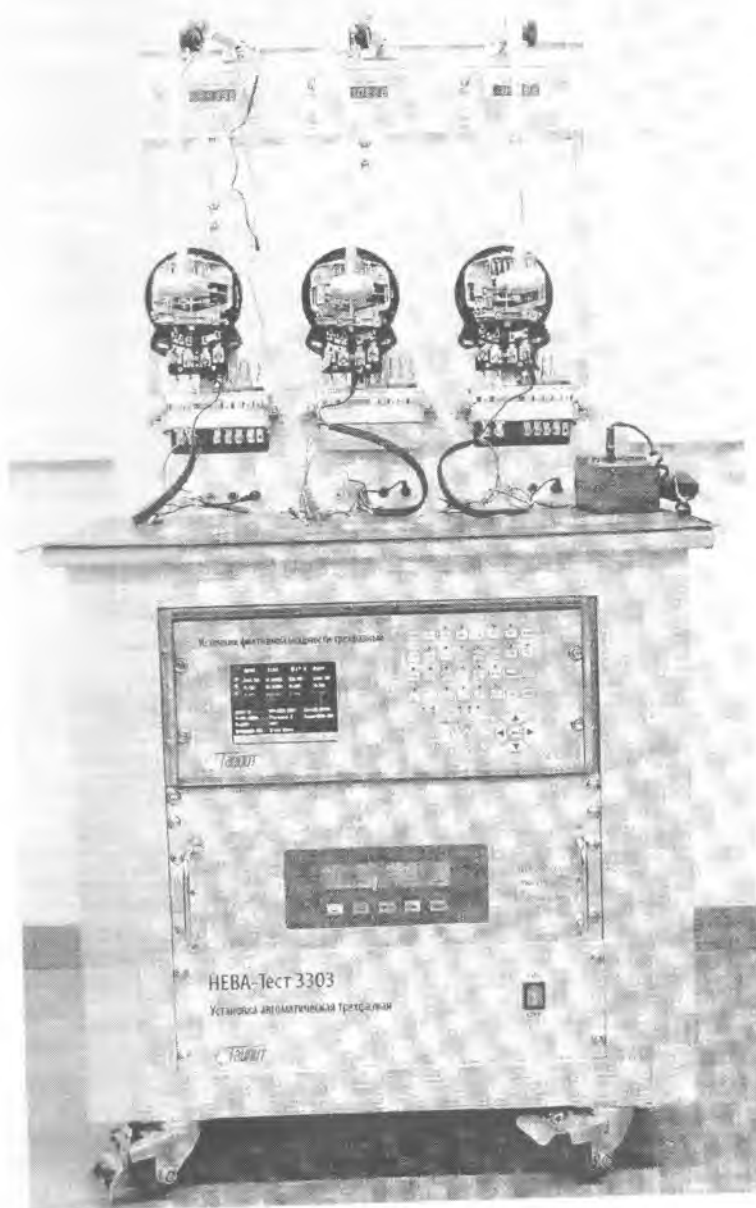
Рис.1 Установка НЕВА-Тест 3303Л
