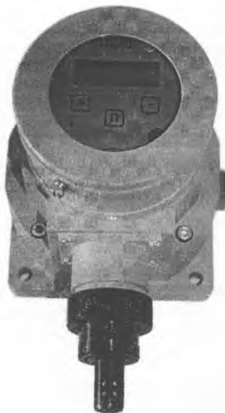
Рисунок 2 – Газоанализатор стационарный со сменными сенсорами взрывозащищенный ССС-903 (исполнение ССС-903 с УПЭС-903 с индикацией), внешний вид.
