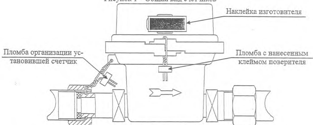
Рисунок 2 – Места пломбировки
