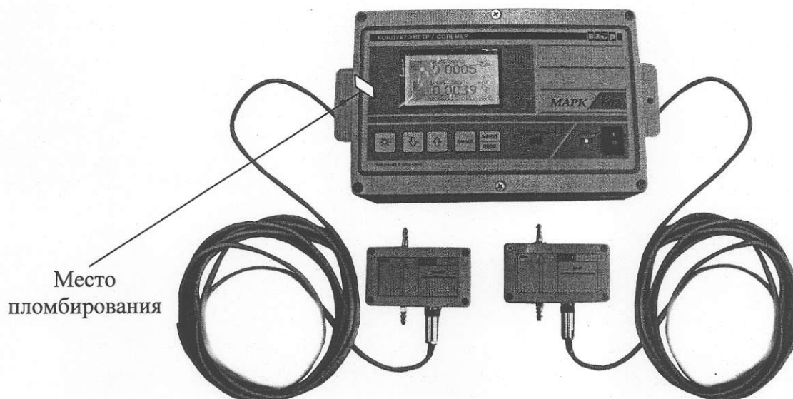
Рисунок – Кондуктометр-солемер МАРК-602 с датчиками проводимости ДП-025С и ДП-2С
