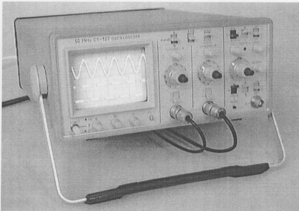
Рисунок 1 - Осциллограф С1-127. Общий вид.
