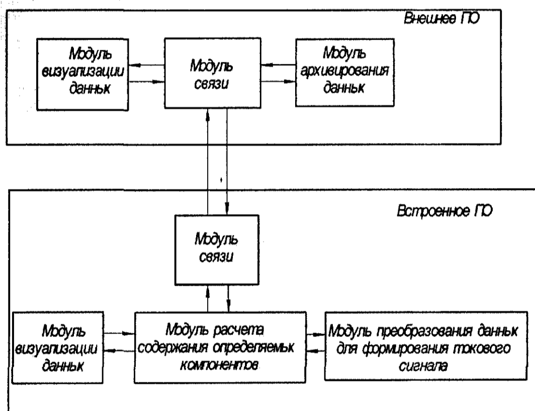
Рисунок 1. Структура ПО.
