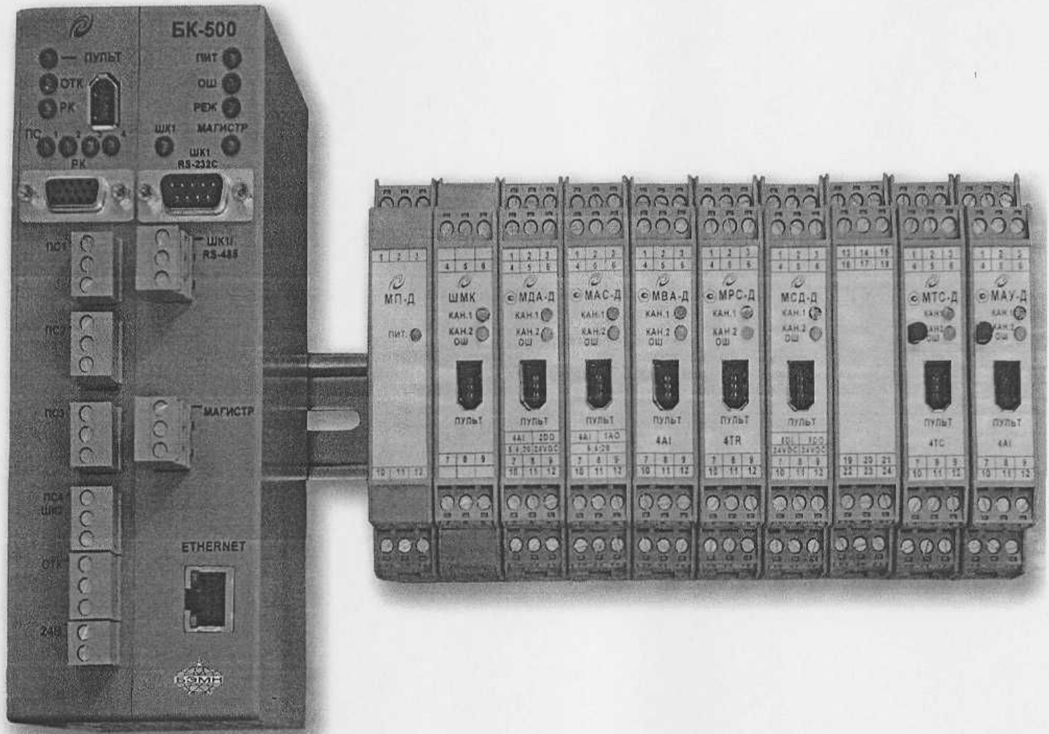
Рисунок 1 – Внешний вид контроллеров
