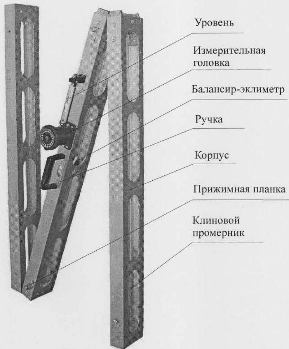
Рисунок 1 – Внешний вид рейки дорожной универсальной РДУ-АНДОР
