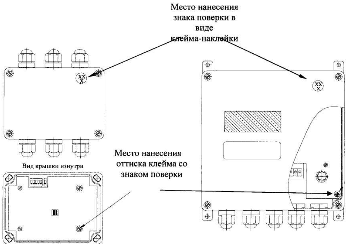
б) исполнение РСМ - 05.05, РСМ - 05.05С, РСМ - 05.07
