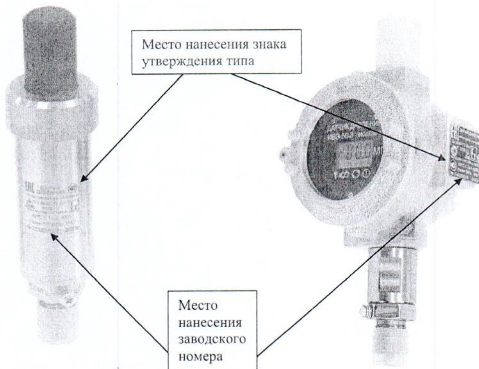
Рисунок 3 – Общий вид датчиков давления ИВЭ-50-3, модель 03
