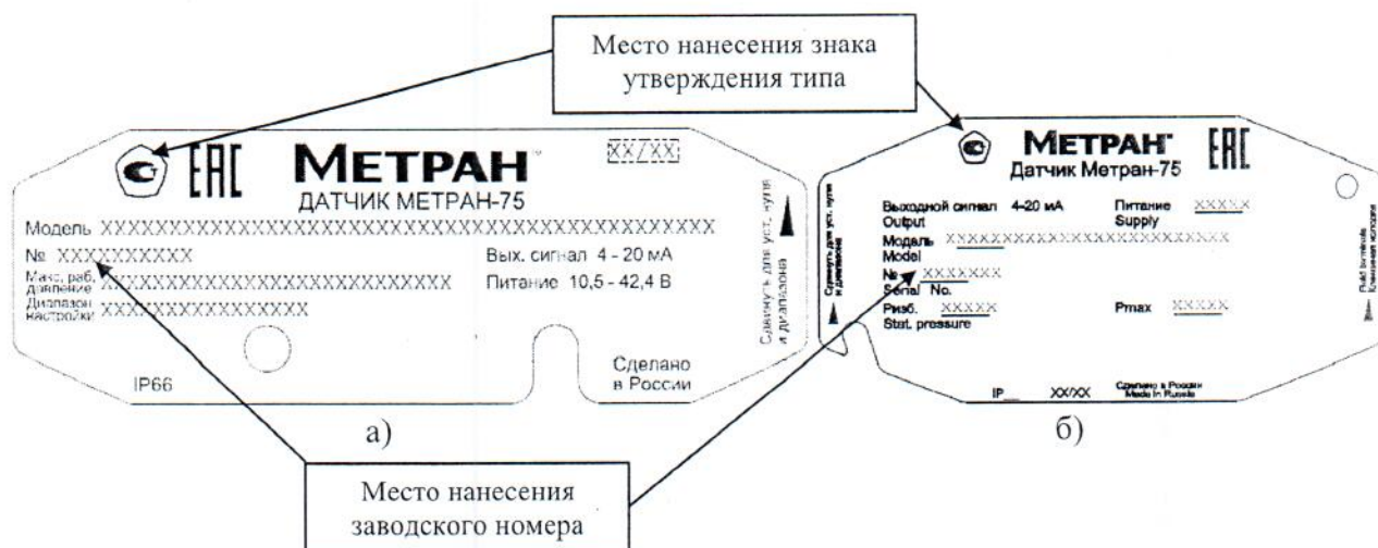
Рисунок 2 – Общий вид (схема) маркировочной таблички для датчиков: а) моделей 75А, 75G; б) моделей 75РА, 75ТА, 75ТG, 75РG, 75СG, 75СD и место нанесения знака утверждения типа и заводского номера
