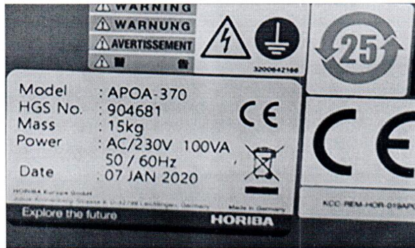
Рисунок 1.2 – Фотография маркировки анализатора озона АРОА-370 № 904681
