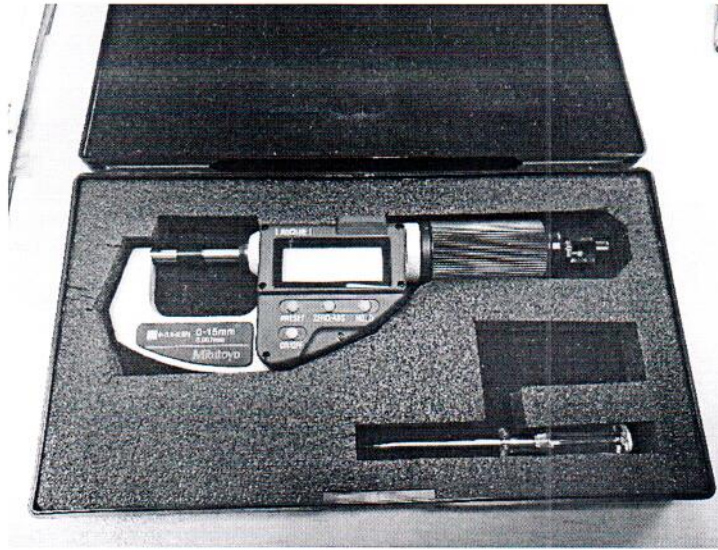
Рисунок 1.1 – Фотография общего вида микрометра Mitutoyo ABSOLUTE серии 227-201-20 № 61051166
