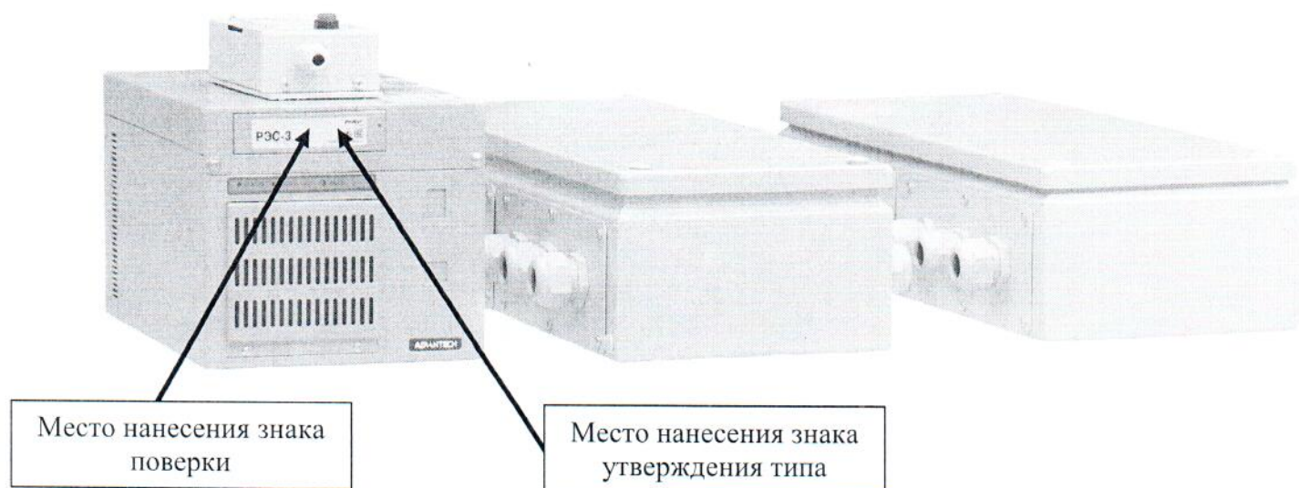
Рисунок 2 – Общий вид регистраторов в стационарном (блочном) исполнении
