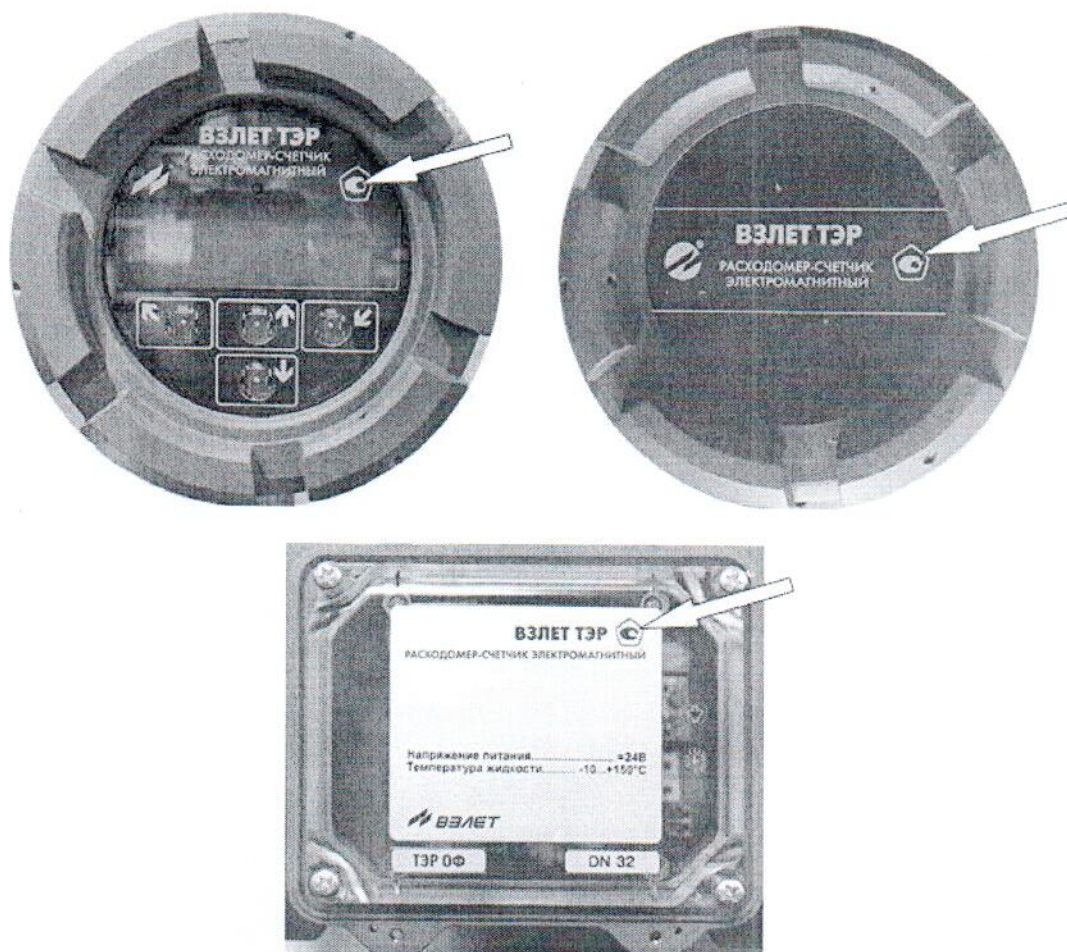
Рисунок 4 – Обозначение места нанесения знака утверждения типа
