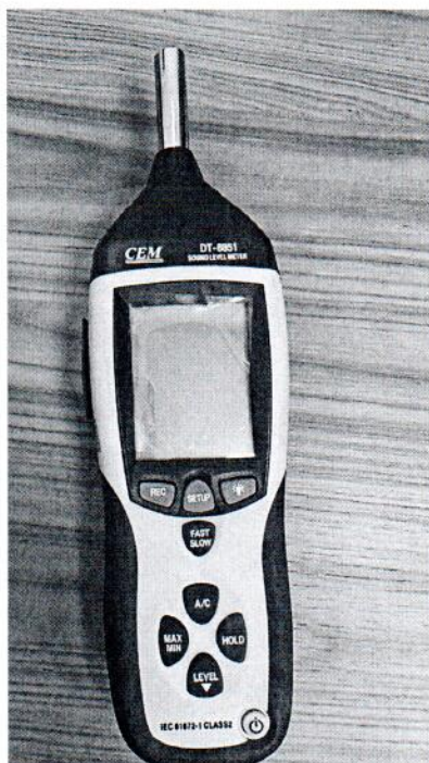
Рисунок 1.1 – Фотография общего вида измерителя уровня звука DT- 8851 № 12044666
