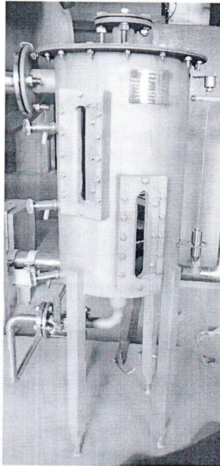
Рисунок 1.1 – Внешний вид мерника ММТ-50 № 9283
