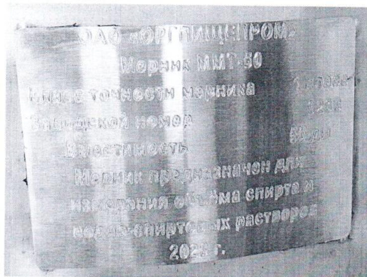
Рисунок 1.2 – Внешний вид маркировочной таблички мерника ММТ-50 № 9283
