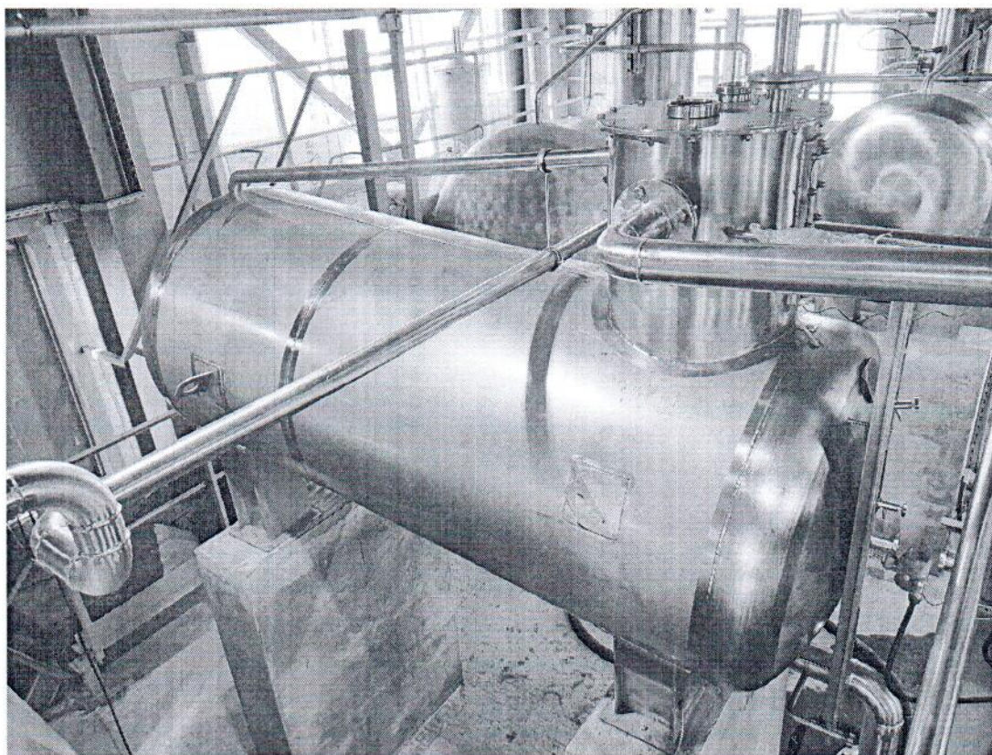
Рисунок 1.1 – Внешний вид мерника металлического технического ММТ-250 № 833
