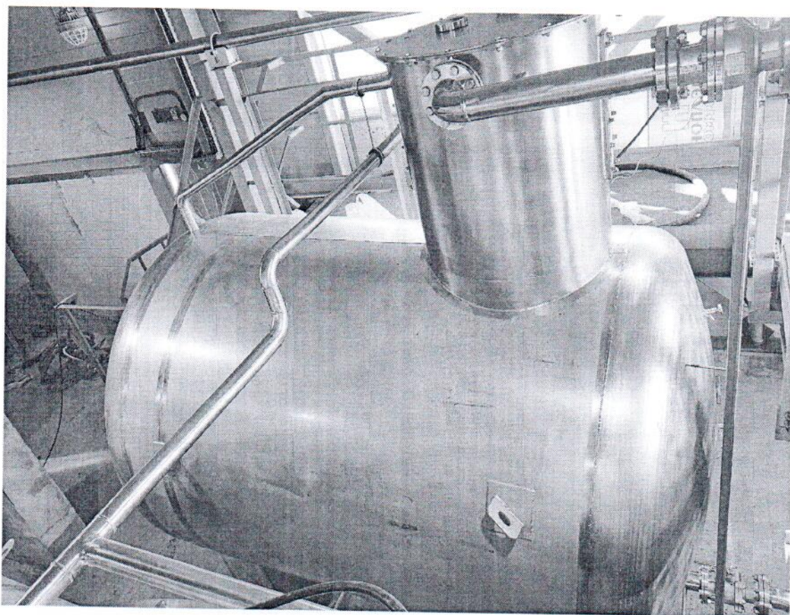
Рисунок 1.1 – Внешний вид мерника металлического технического ММТ-1000 № 839
