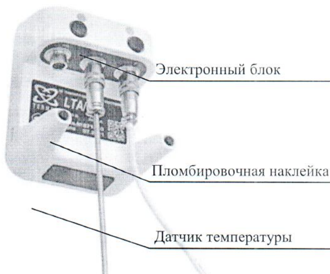
Рисунок 1 – Внешний вид термометра с дискретными входом/выходами и двумя каналами измерений температуры: канал 1 – датчик с разъемным соединением, подключенный непосредственно к электронному блоку; канал 2 – датчик с разъемным соединением, подключенный к электронному блоку с помощью кабеля-удлинителя
