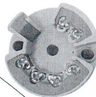
Рисунок 1.3 – VME-100-2, VME-101-2, VME-Exi-102-2
