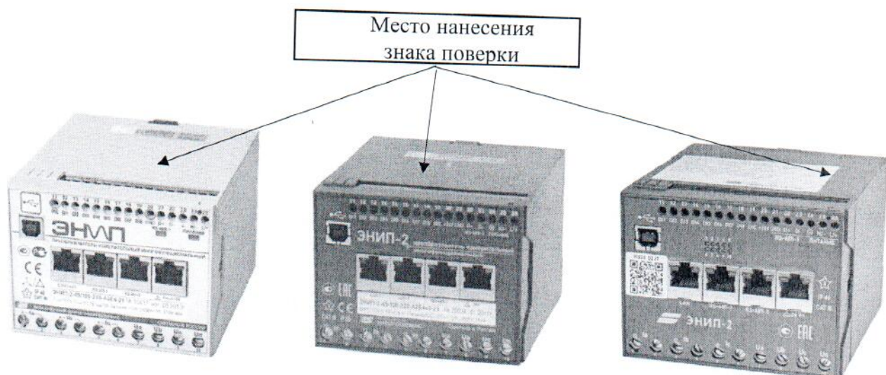
Рисунок 1 – Общий вид преобразователей модификации ЭНИП-2-...-X1
