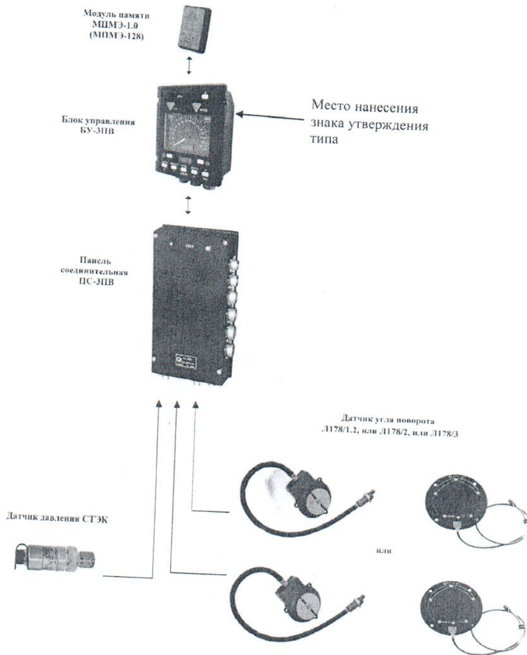
Рисунок 5 – Общий вид КПД-ЗПВ
