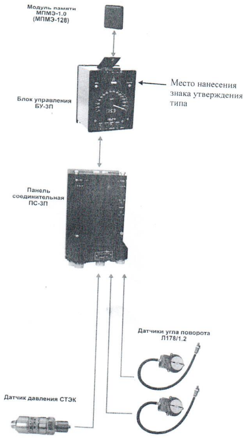
Рисунок 2 – Общий вид КПД-ЗП
