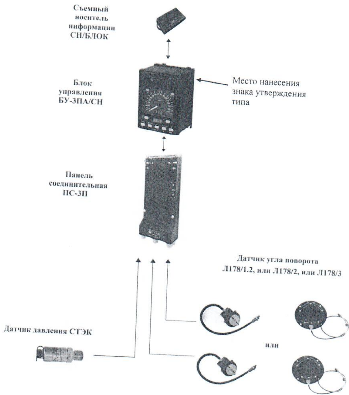
Рисунок 4 – Общий вид КПД-3ПА/СН
