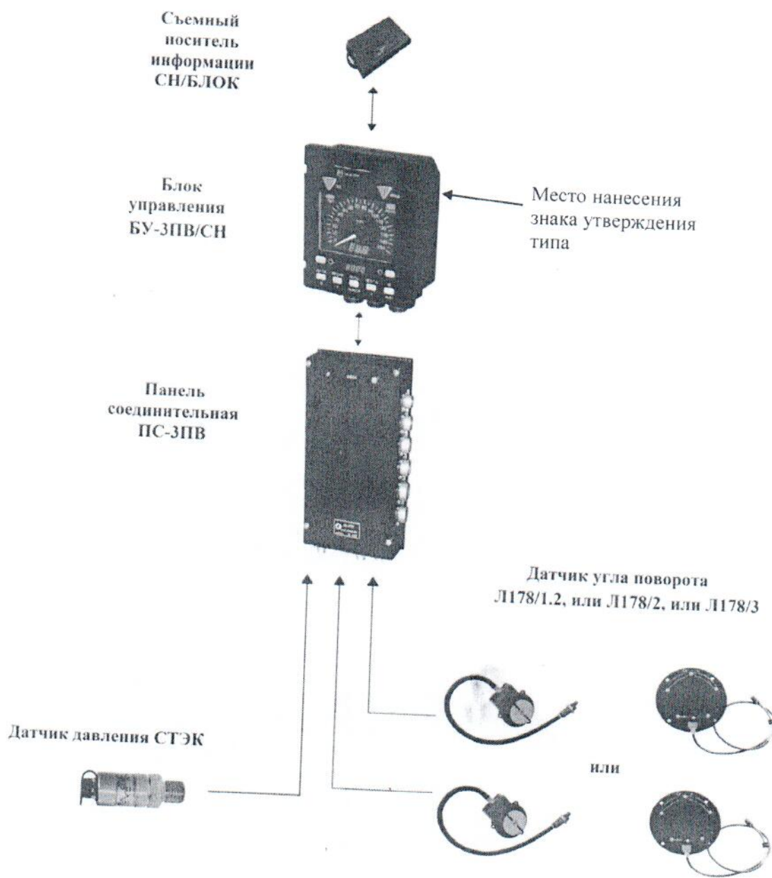
Рисунок 6 – Общий вид КПД-3ПВ/СН
