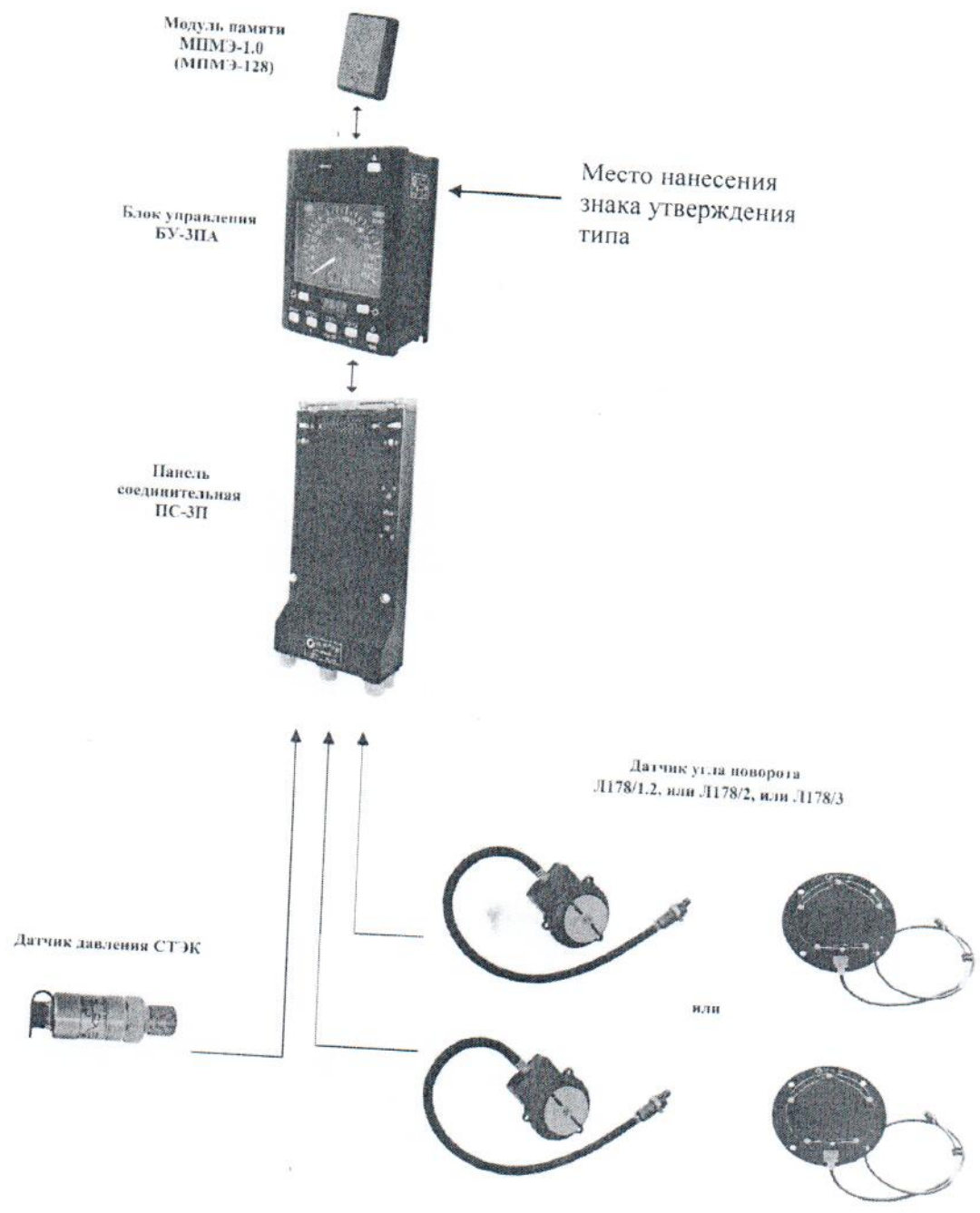
Рисунок 3 – Общий вид КПД-ЗПА
