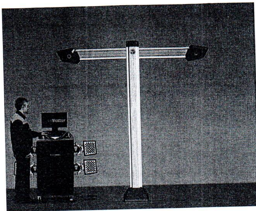
Рисунок 6 – модификация 7202 (Корпус камер тип Т)
