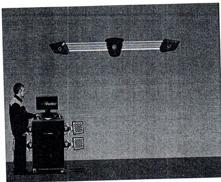
Рисунок 7 – модификация 7202 (Корпус камер тип К)
