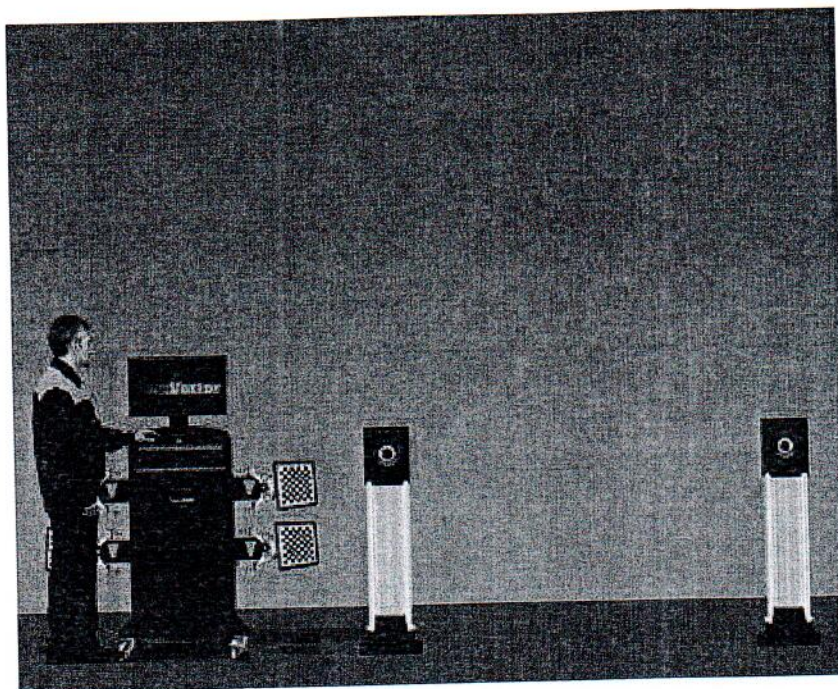
Рисунок 8 – модификация 7202 (Корпус камер тип М)
