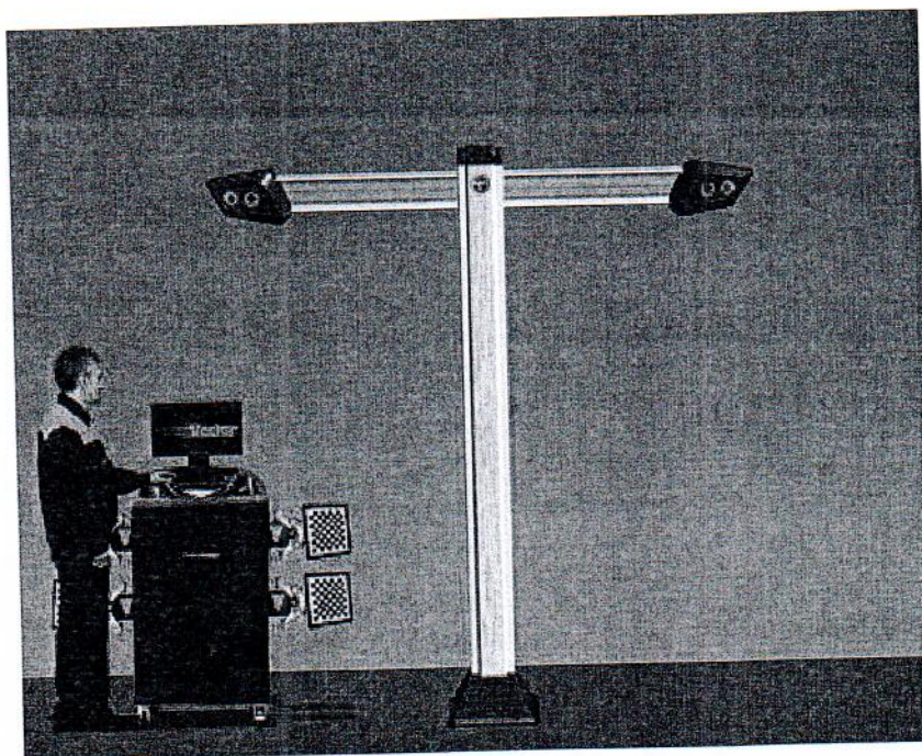
Рисунок 9 – модификация V 7204 T A (Корпус камер тип Т)
