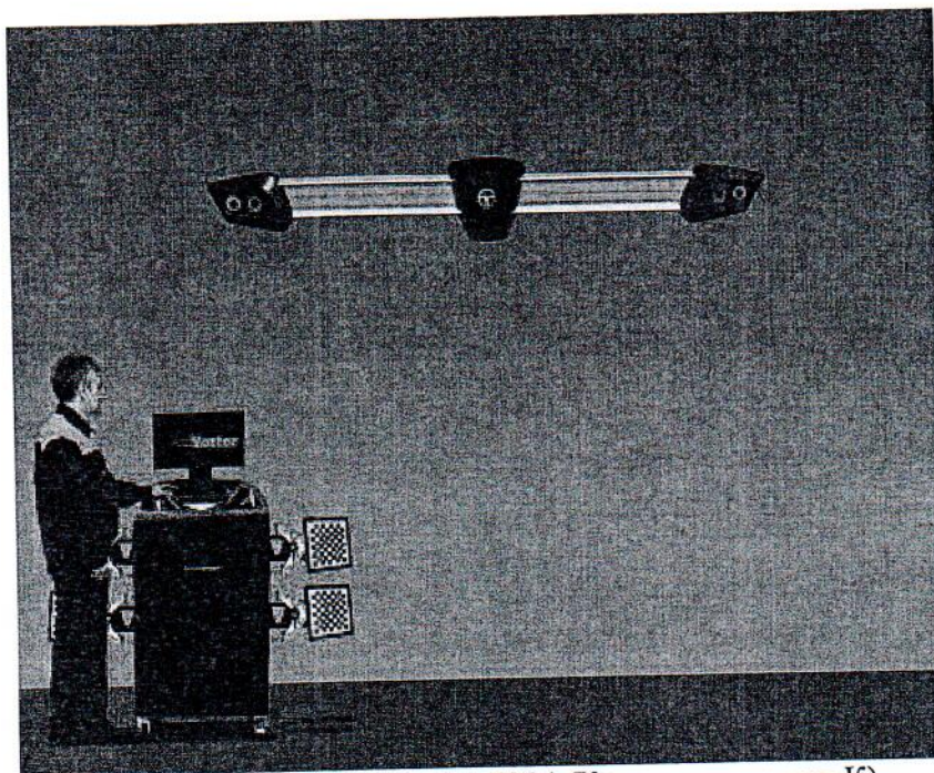
Рисунок 14 – модификация 7204 (Корпус камер тип К)
