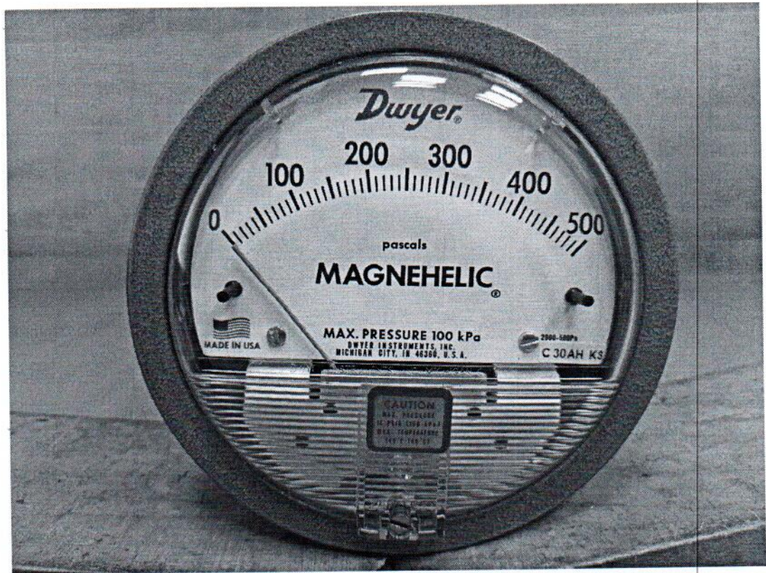
Рисунок 1.1 – Фотография общего вида манометра дифференциального показывающего Magnehelic 2000-500PA № 4CFA-EUMS-JWBP-2RHX
