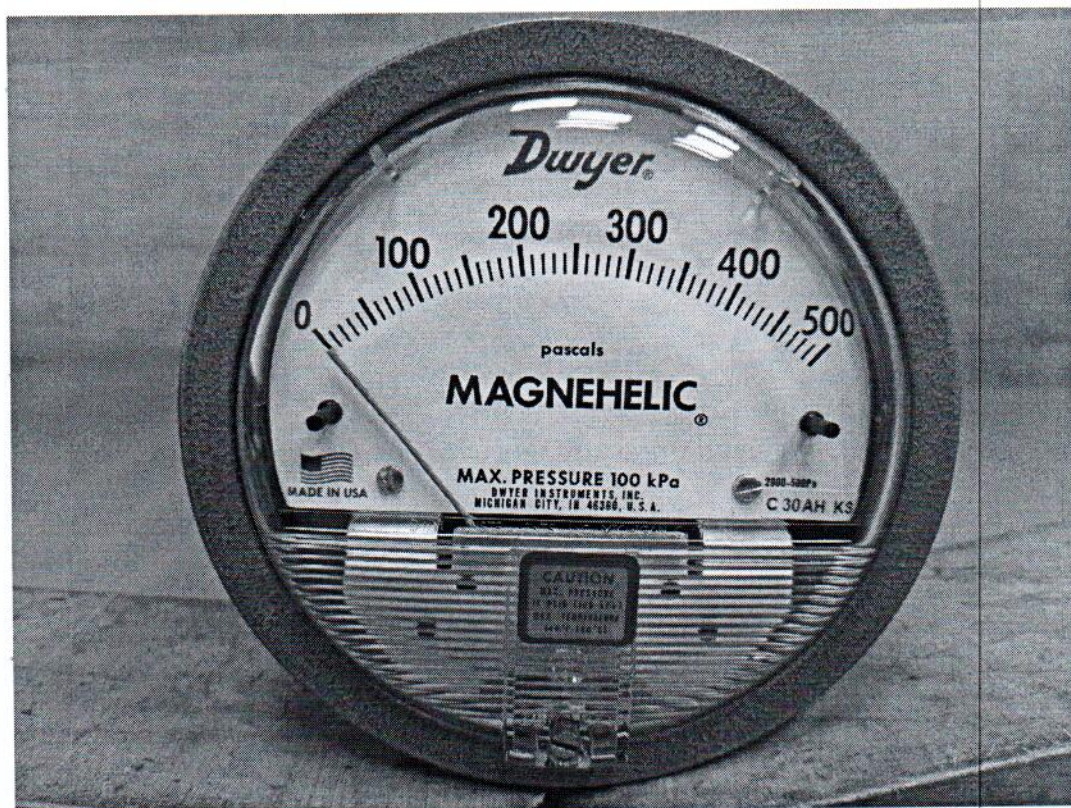
Рисунок 1.1 – Фотография общего вида манометра дифференциального показывающего Magnehelic 2000-500PA № 4CFA-F6EV-TVV6-ZLSF
