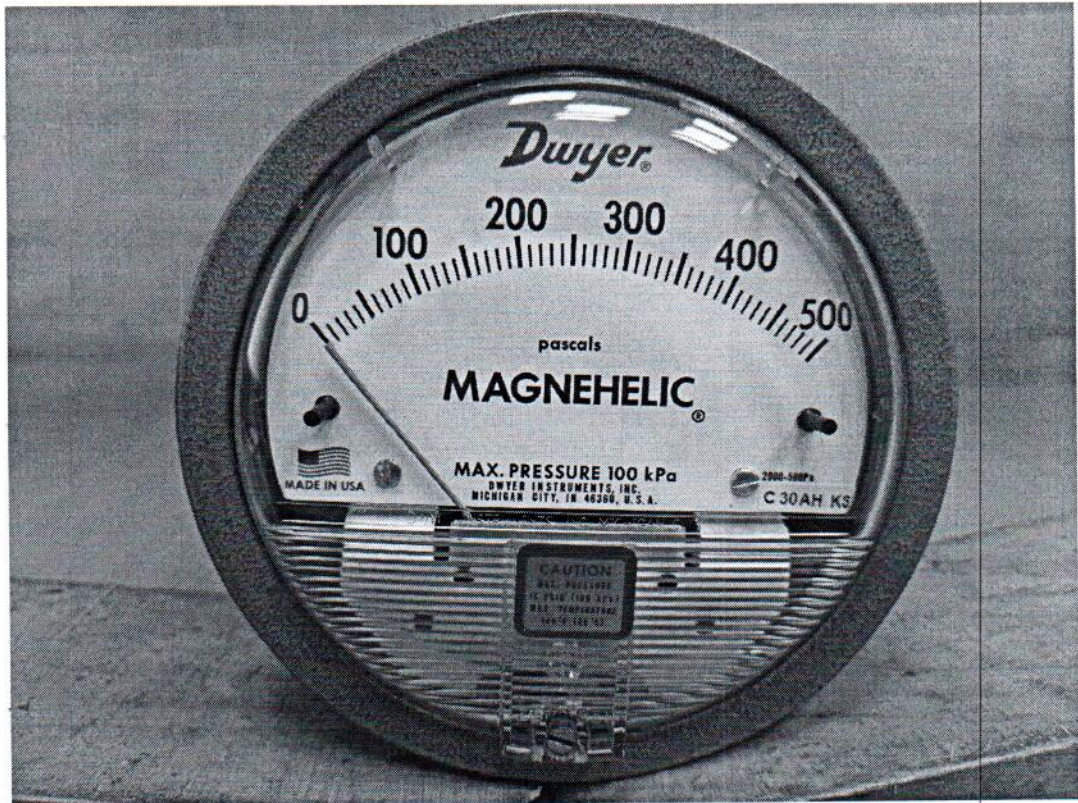
Рисунок 1.1 – Фотография общего вида манометра дифференциального показывающего Magnehelic 2000-500PA № 4CFA-E2N1-ZNPQ-82IU
