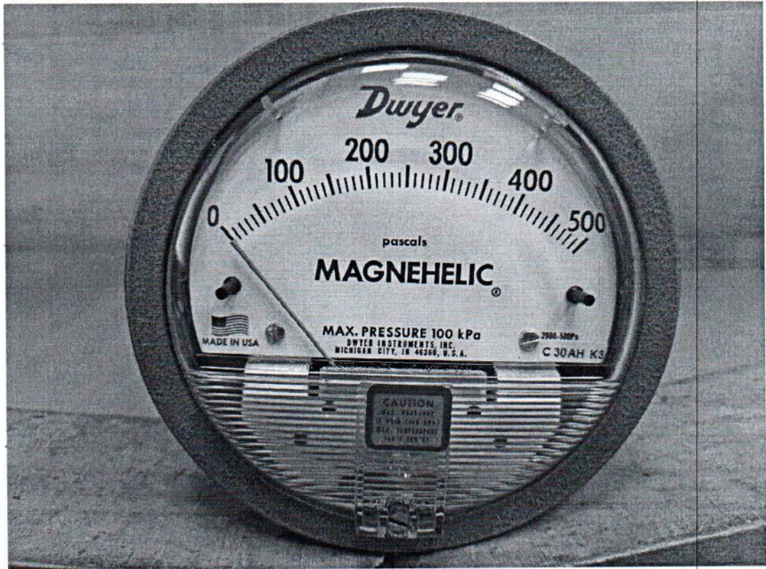
Рисунок 1.1 – Фотография общего вида манометра дифференциального показывающего Magnehelic 2000-500PA № 4CFA-EEVQ-LFDZ-9VH2
