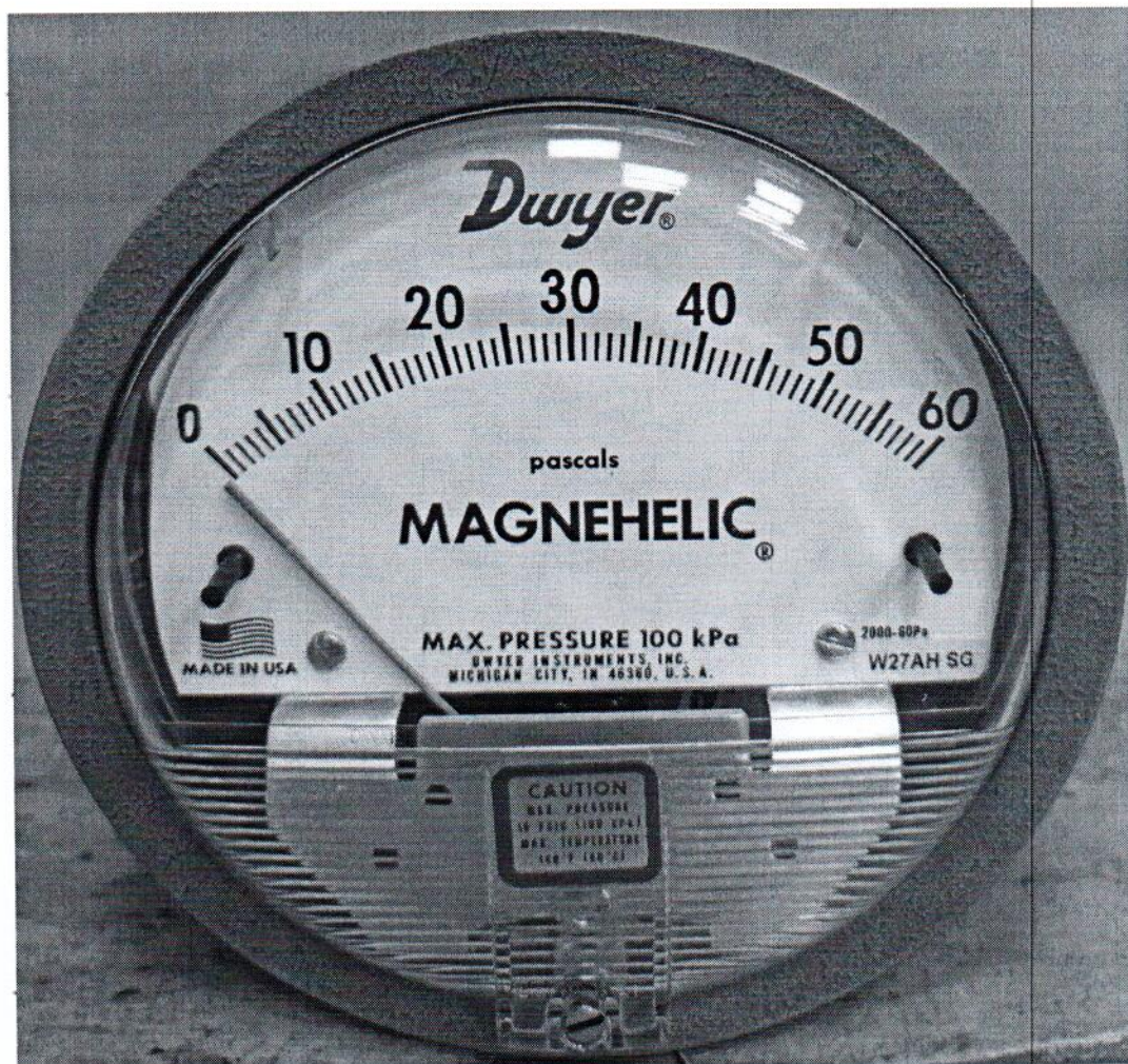
Рисунок 1.1 – Фотография общего вида манометра дифференциального показывающего Magnehelic 2000-60РА № 161222СК-40
