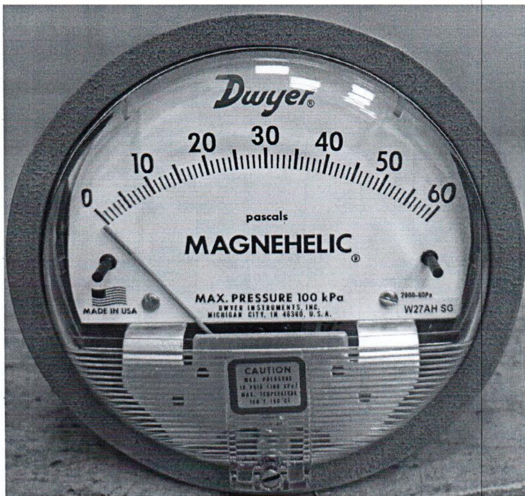
Рисунок 1.1 – Фотография общего вида манометра дифференциального показывающего Magnehelic 2000-60PA № 161222СК-38
