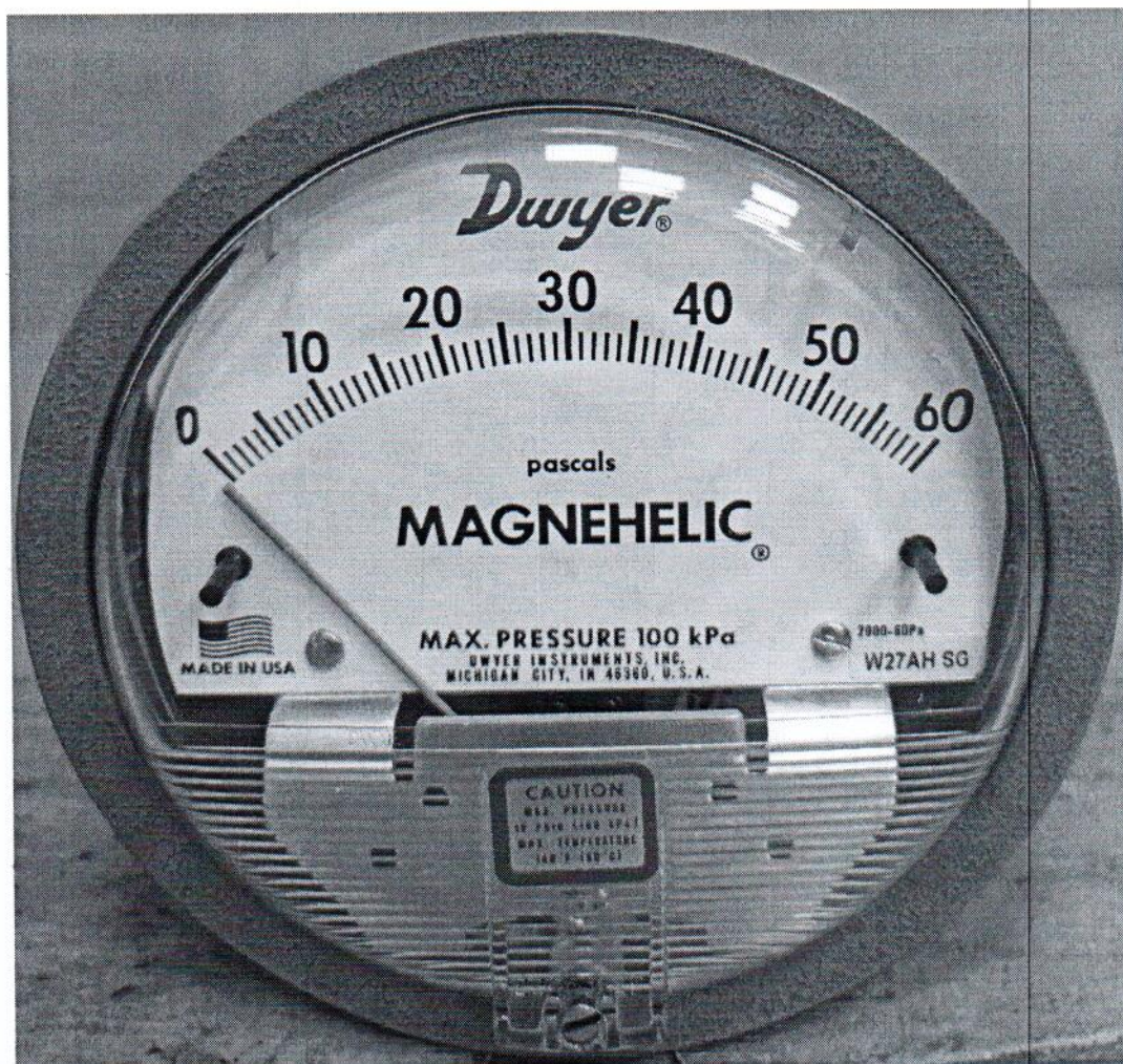
Рисунок 1.1 – Фотография общего вида манометра дифференциального показывающего Magnehelic 2000-60РА № 161222СК-29
