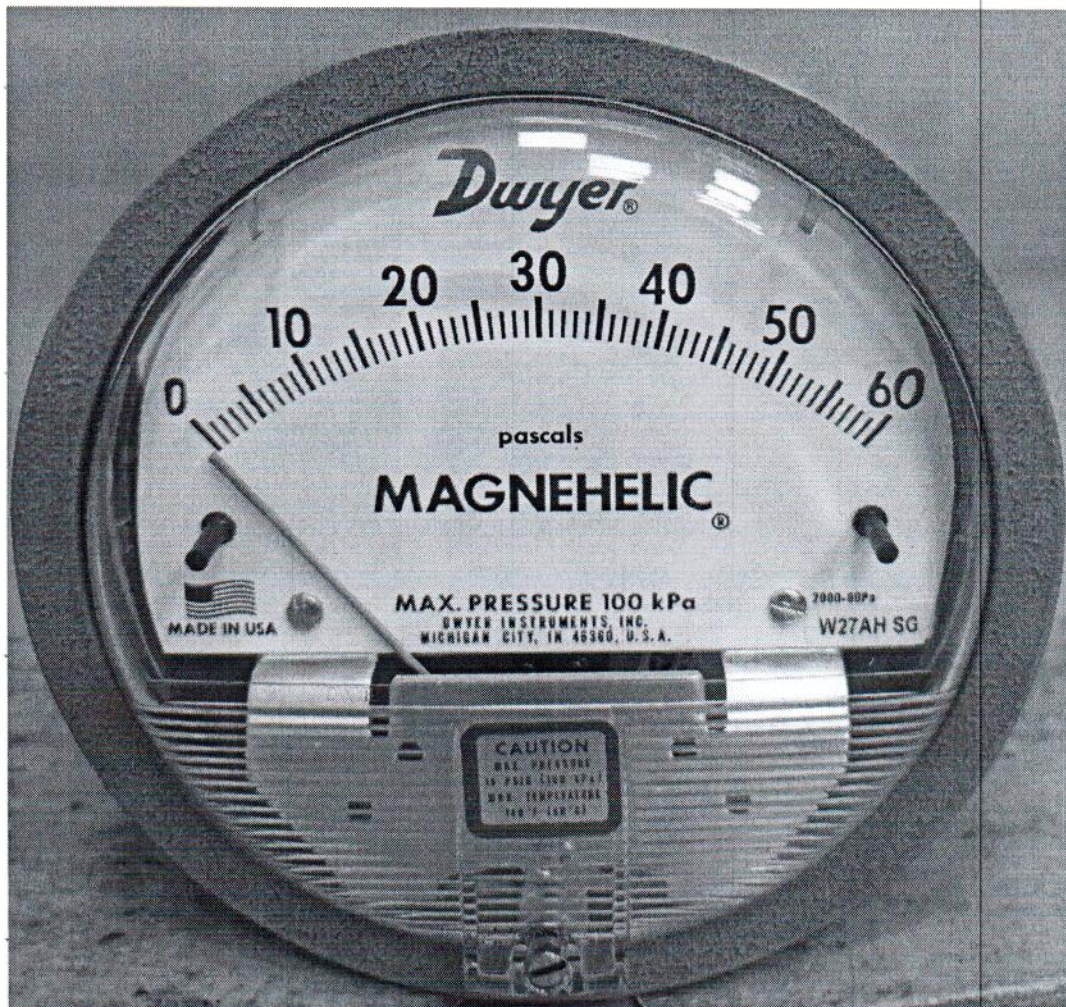
Рисунок 1.1 – Фотография общего вида манометра дифференциального показывающего Magnehelic 2000-60PA № 161222СК-27
