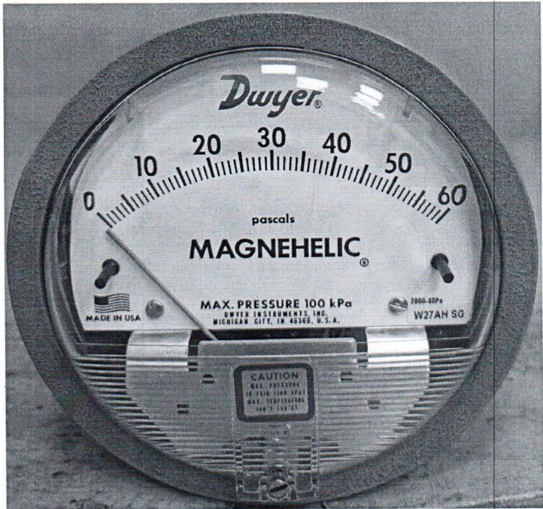
Рисунок 1.1 – Фотография общего вида манометра дифференциального показывающего Magnehelic 2000-60РА № 161222СК-23
