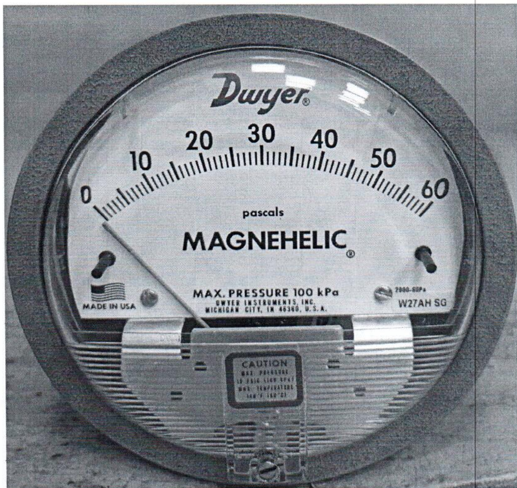
Рисунок 1.1 – Фотография общего вида манометра дифференциального показывающего Magnehelic 2000-60PA № 161222СК-21
