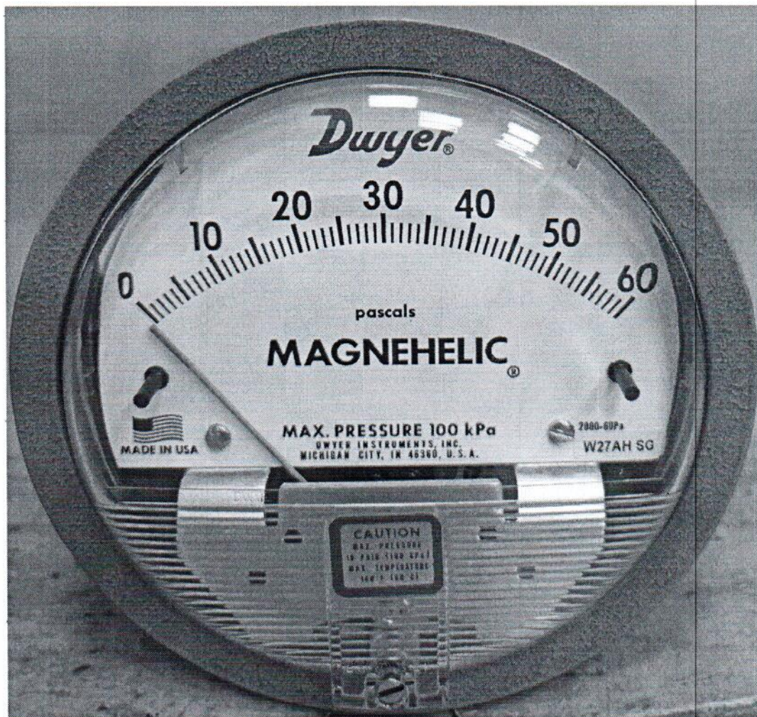
Рисунок 1.1 – Фотография общего вида манометра дифференциального показывающего Magnehelic 2000-60PA № 161222СК-20
