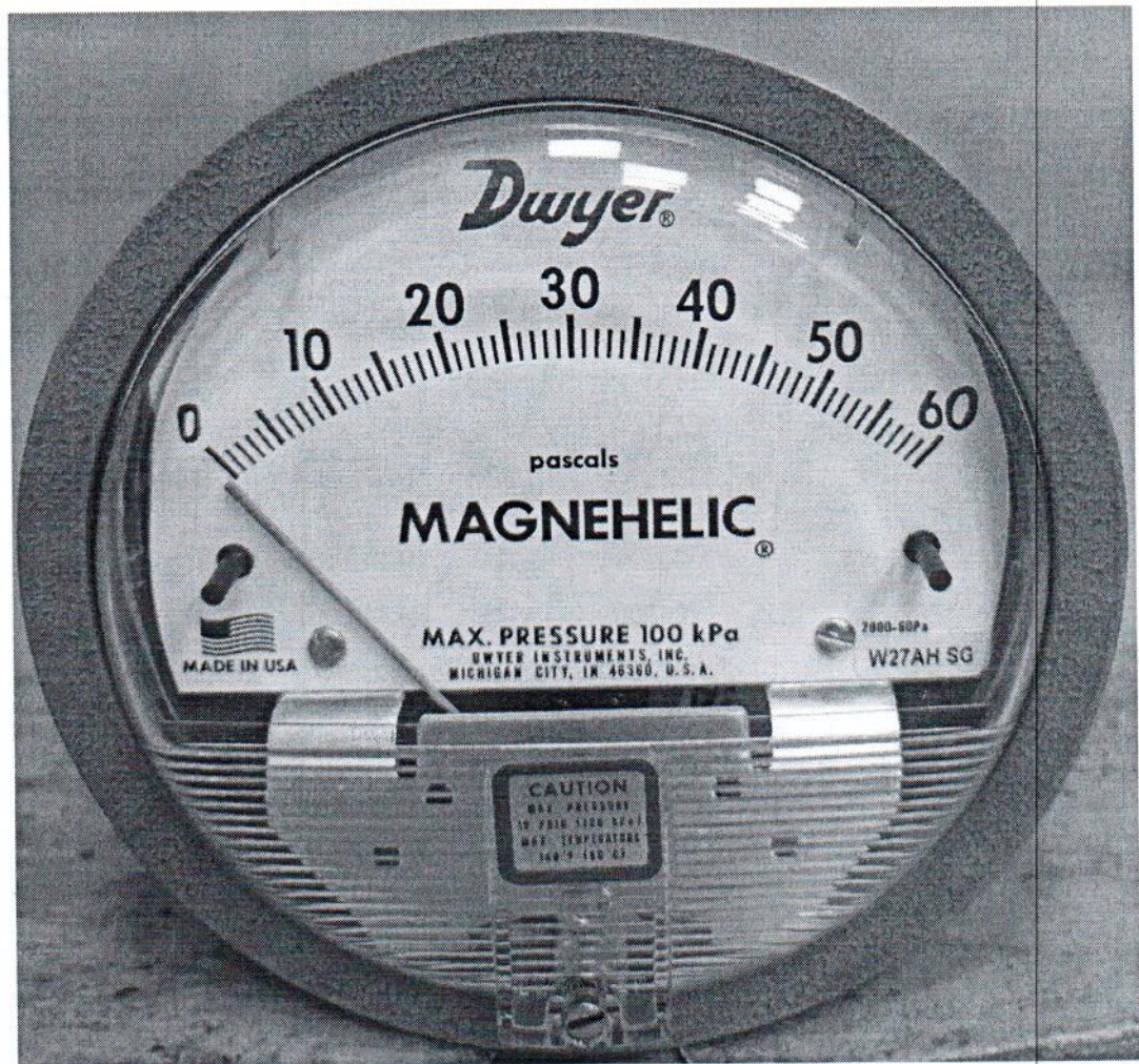
Рисунок 1.1 – Фотография общего вида манометра дифференциального показывающего Magnehelic 2000-60PA № 161222СК-14
