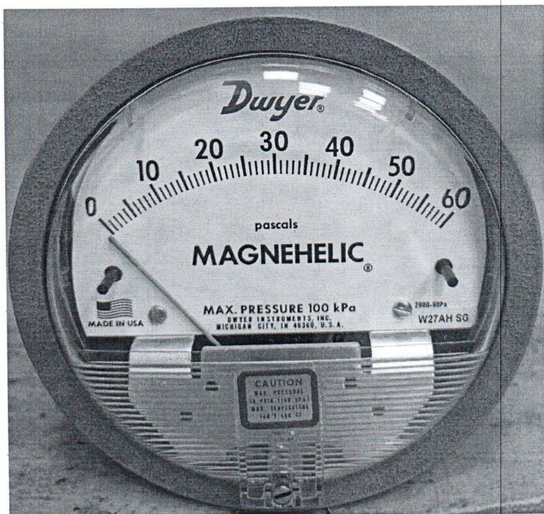
Рисунок 1.1 – Фотография общего вида манометра дифференциального показывающего Magnehelic 2000-60PA № 161222СК-09
