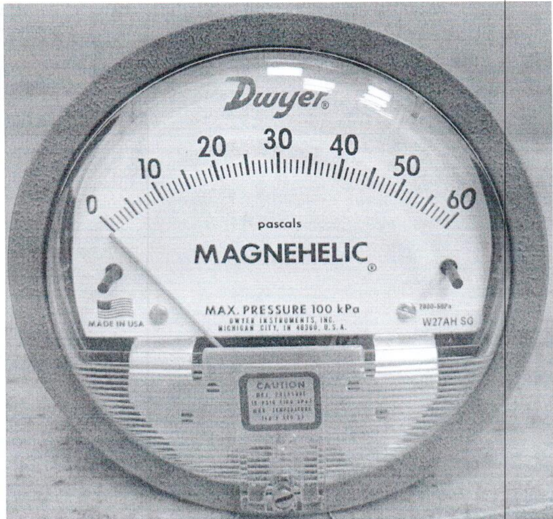
Рисунок 1.1 – Фотография общего вида манометра дифференциального показывающего Magnehelic 2000-60PA № 161222СК-01
