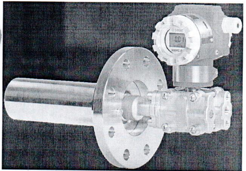
ЭМИС-БАР 163; ЭМИС-БАР 164
