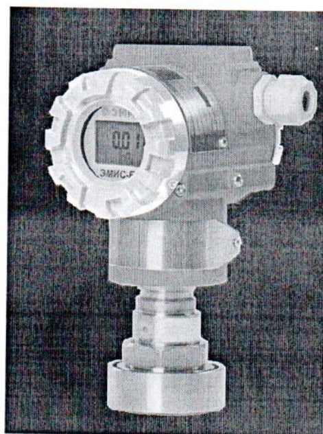
ЭМИС-БАР 103; ЭМИС-БАР 123
