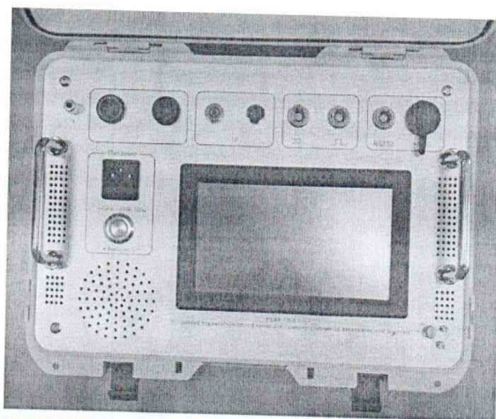
Рисунок 2 – Панель управления установки переносной однофазной для поверки счетчиков электрической энергии НЕВА-Тест 3101
