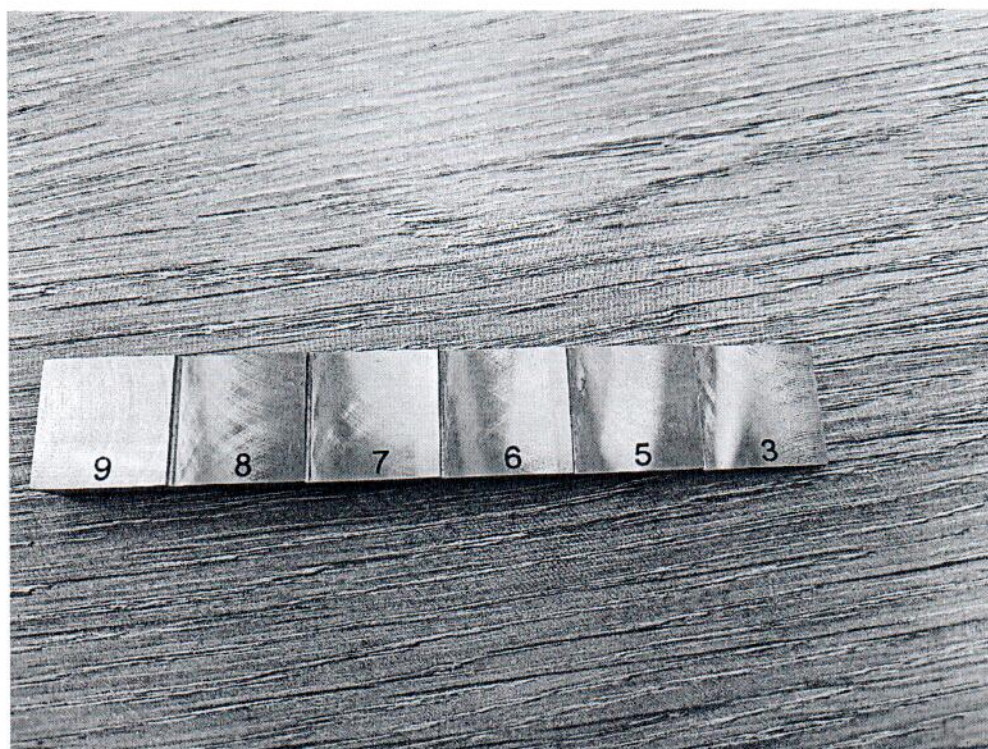
Рисунок 1.1 – Фотография общего вида настроечного образца типа «Ступенька» № 2308547
